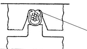
Obermatritze und die sich einrollenden Crimphülsenflanken zwingen das abisolierte Leiterende in den Crimphülsenboden The indenter and the rolling up crimp flanks force the stripped conductor end into the base of the crimp barrel
