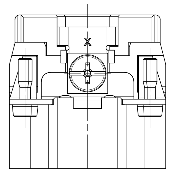
C146 EE für gedrehte Crimpkontakte for turned crimp contacts
