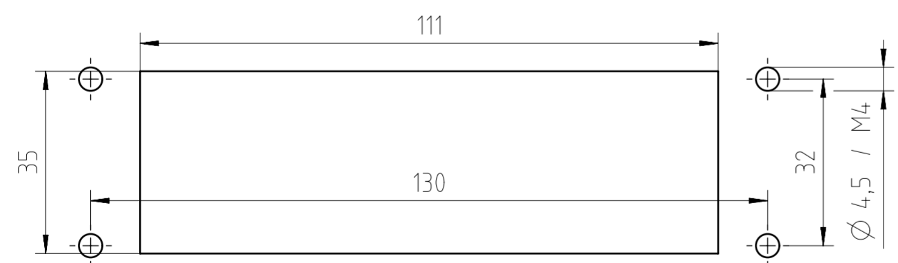
Montageausschnitt Panel cut-out:
