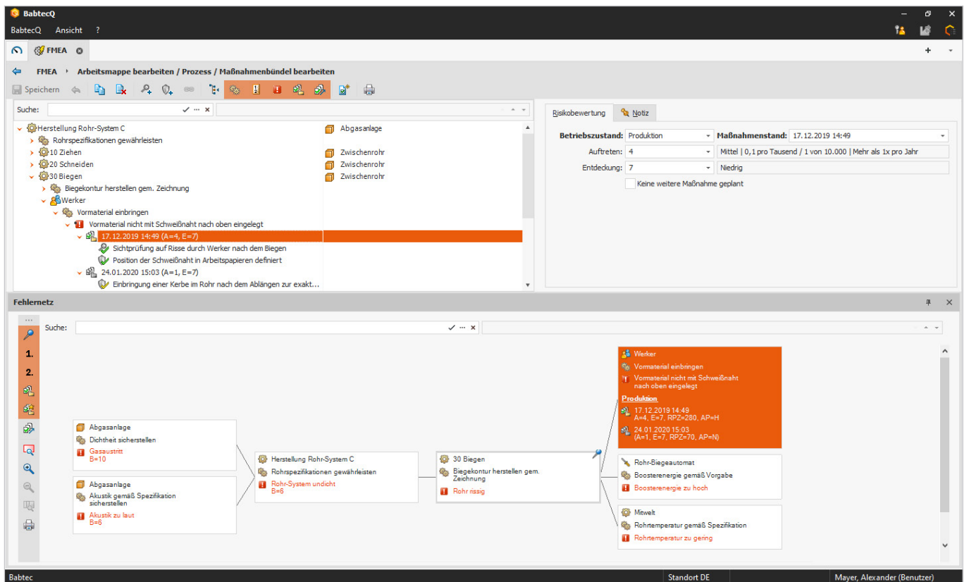
Struktur und Fehlernetz einer Prozess-FMEA
